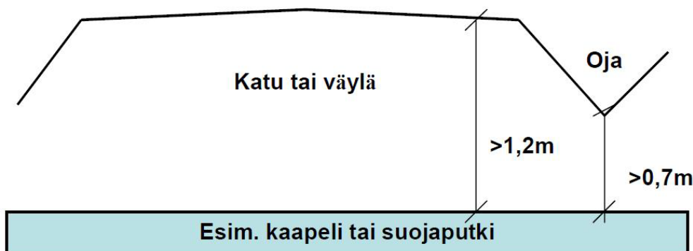
Kuva 1. Minimipeittosyvyydet
