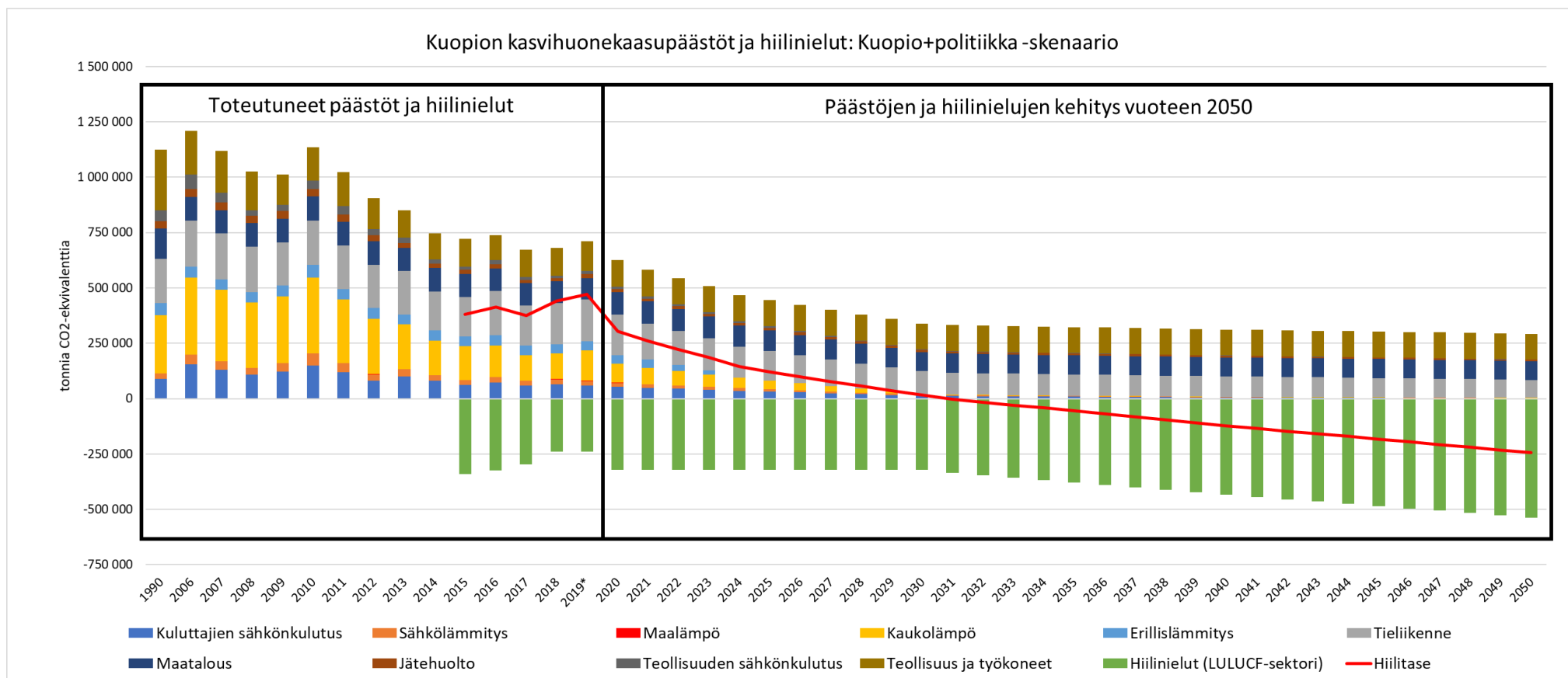
Kuva 4-6. Kuopion kaupungin toteuttamien ja politiikkaskenaarion mukaisten toimenpiteiden mukainen päästöjen ja hiilinielujen kehitys Kuopiossa vuoteen 2050. Päästövähennystarve vuonna 2030 on noin 16 000 tonnia CO 2 -ekv. ja hiilineutraali tilanne saavutetaan noin vuonna 2031.
