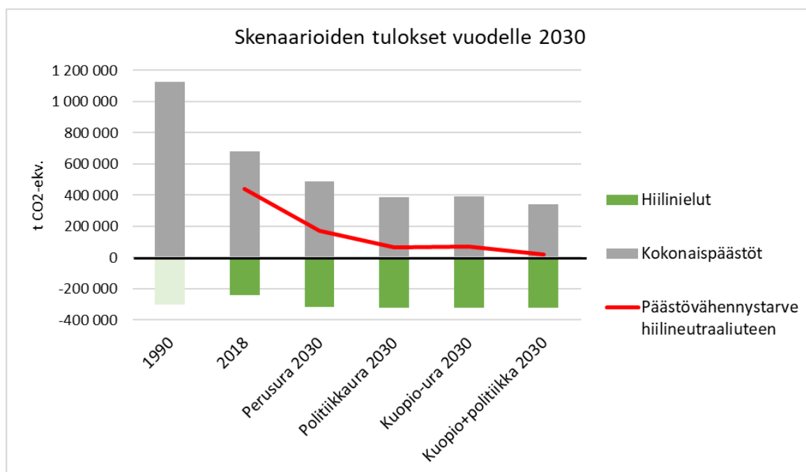
Kuva 4-7 Kokonaispäästöjen ja hiilinielujen muutos eri skenaariossa sekä päästövähennystarve hiilineutraaliuden saavuttamiseksi vuoteen 2030. Vuoden 1990 hiilinieluista ei ole tietoa.
