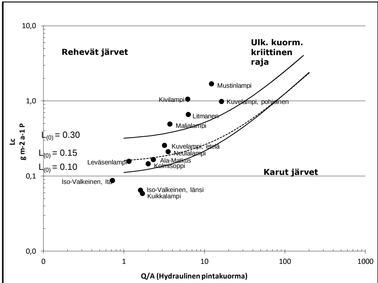
Kuva 2. Lampien A-N ulkoinen kuormitus Vollenweiderin mallin (1975) mukaan.
