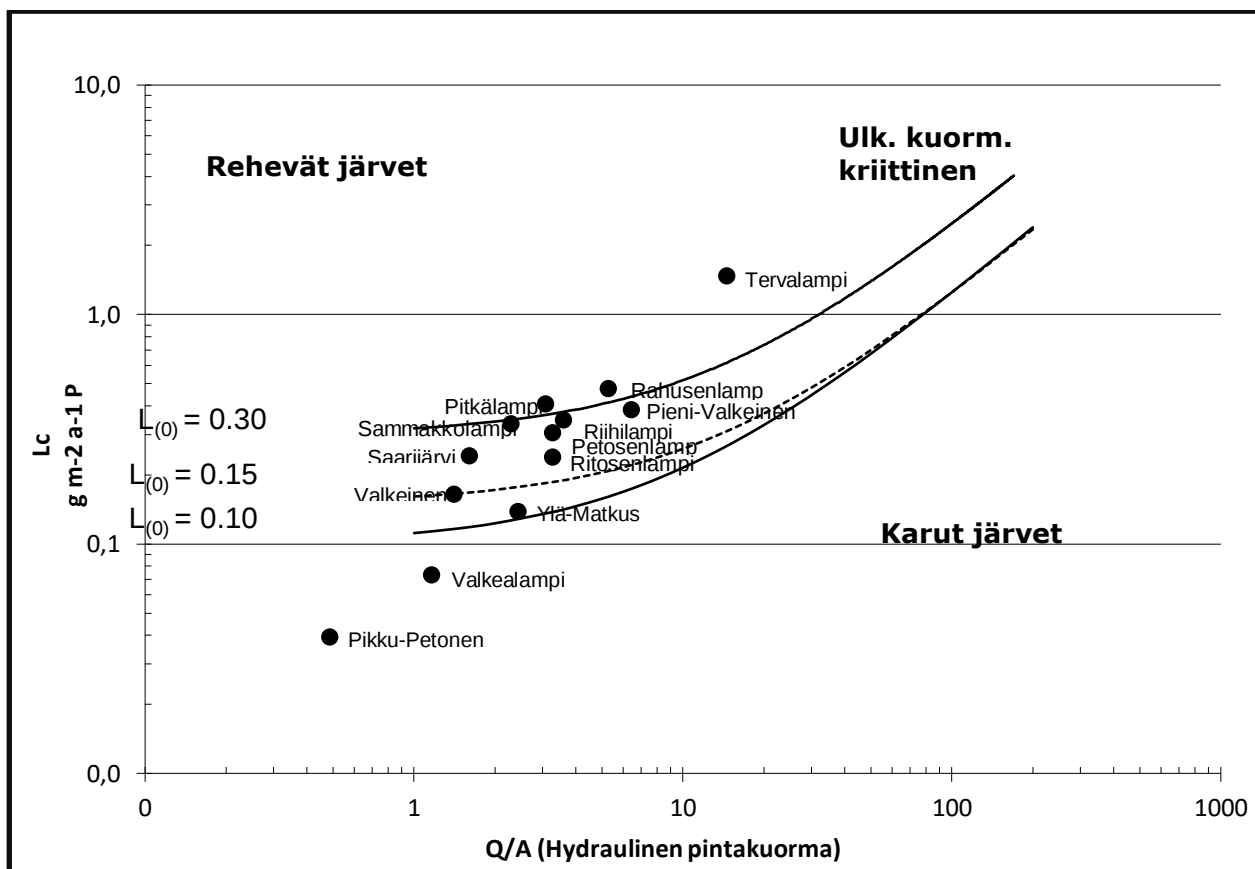
Kuva 3. Lampien P-Y ulkoinen kuormitus Vollenweiderin mallin (1975) mukaan.
