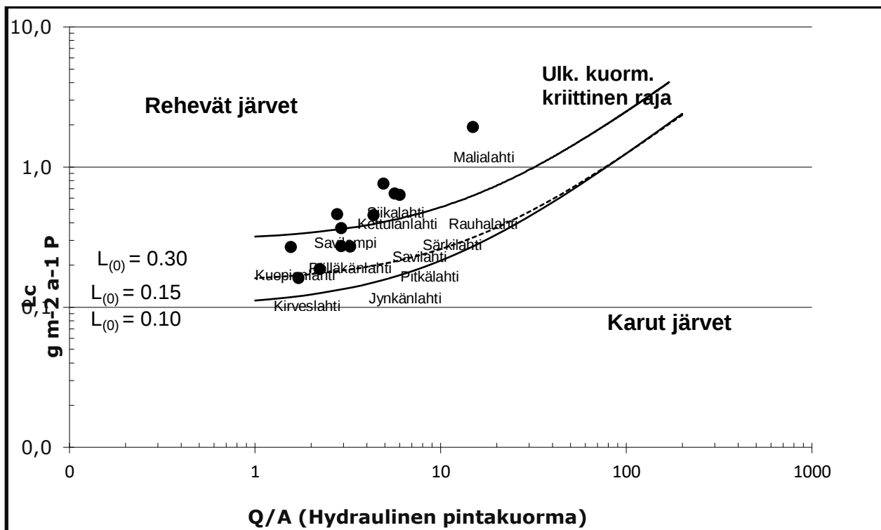
Kuva 4. Lahtien ulkoinen kuormitus Vollenweiderin mallin (1975) mukaan.
