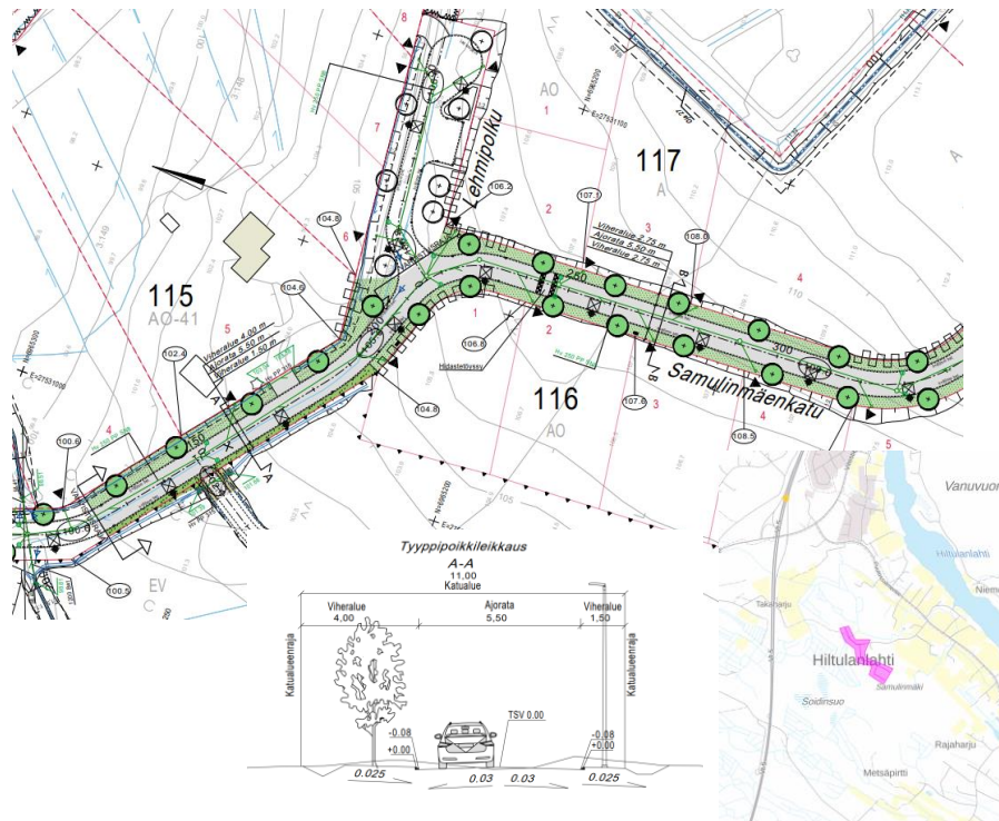
Kuvaote Samulinmäenkadun asemapiirustuksesta ja tyyppipoikkileikkauksesta
