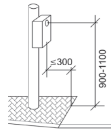
Suojatien painonappipylväs.
